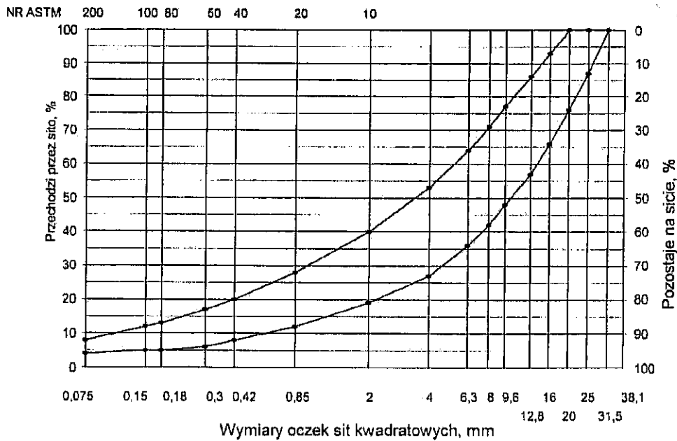
Rys. 2. Krzywe graniczne uziarnienia mieszanki mineralnej BA od 0 do 25mm do podbudowy nawierzchni drogi o obciążeniu ruchem KR 2
