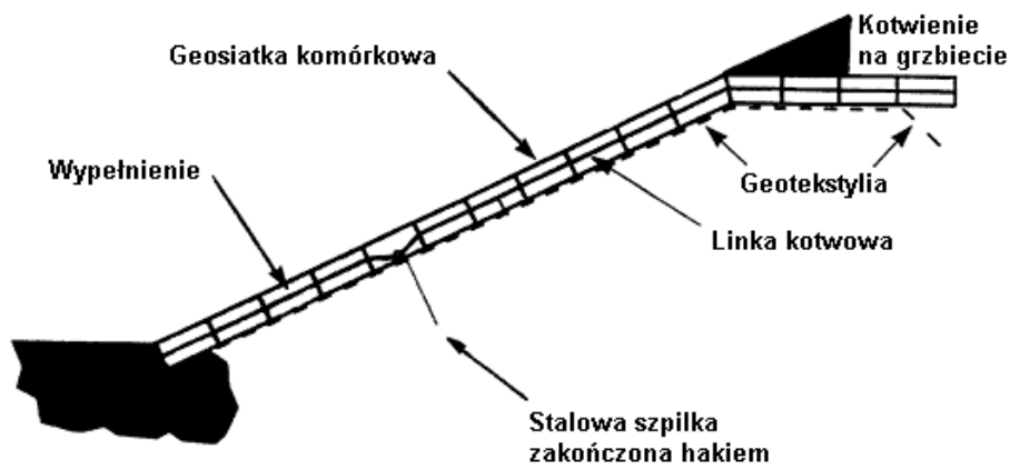
Rys. 7. Umocnienie skarpy geosiatką komórkową
