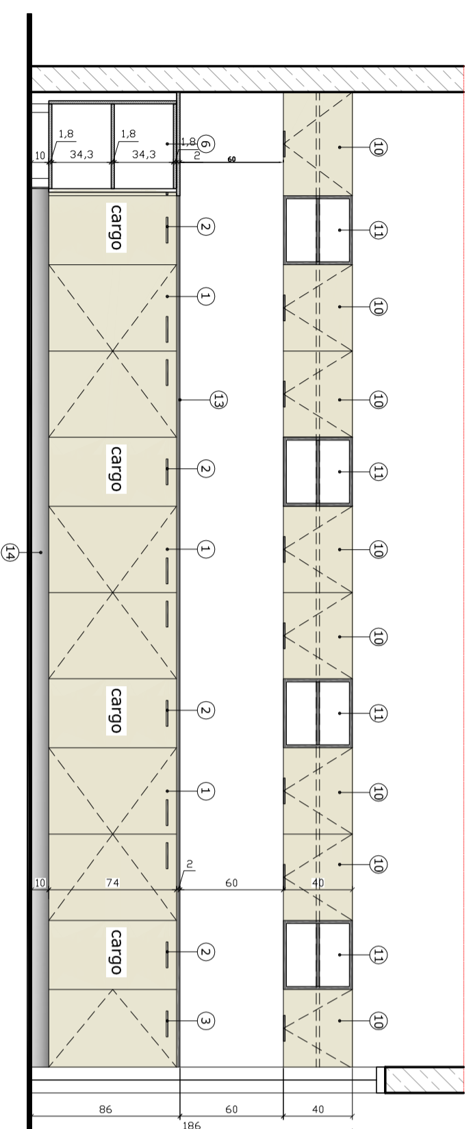
WIDOK A-A (ZCH1)
