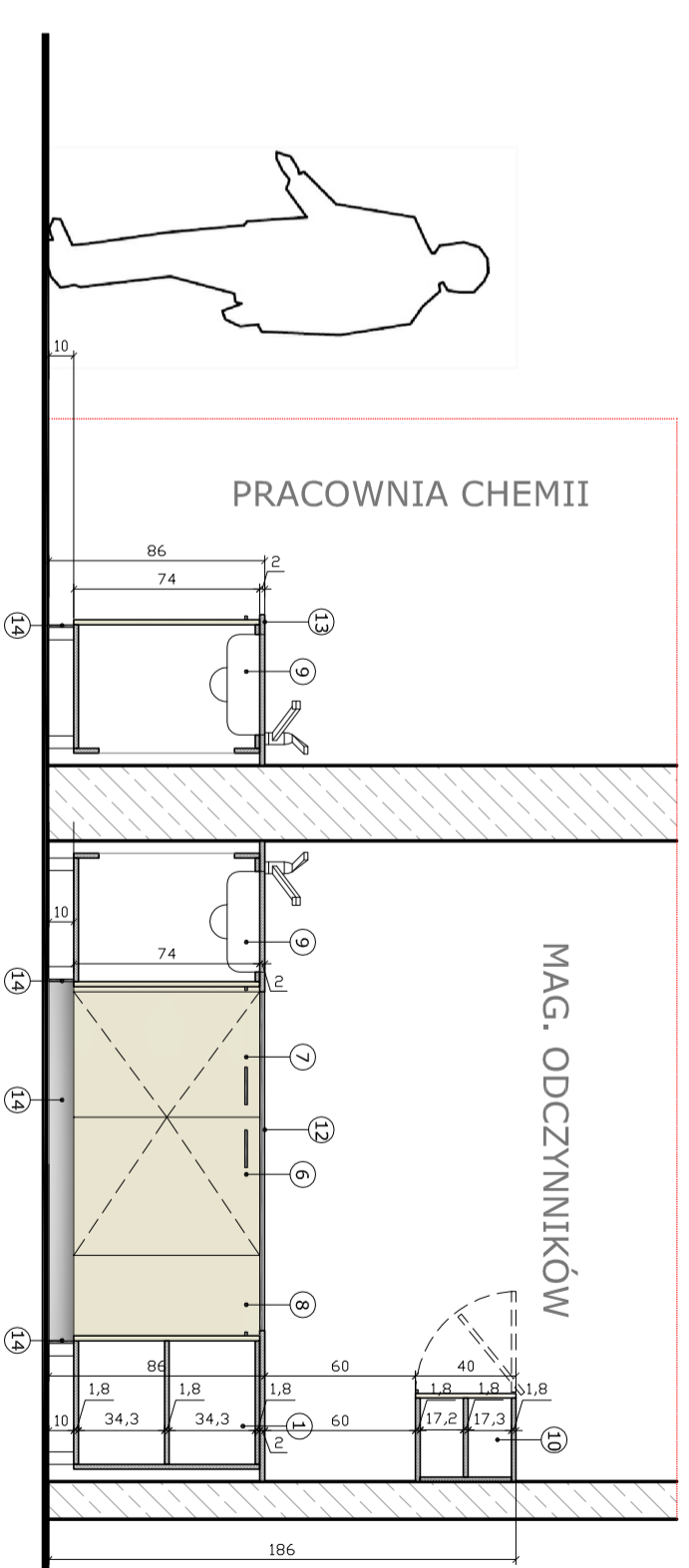
WIDOK C-C
