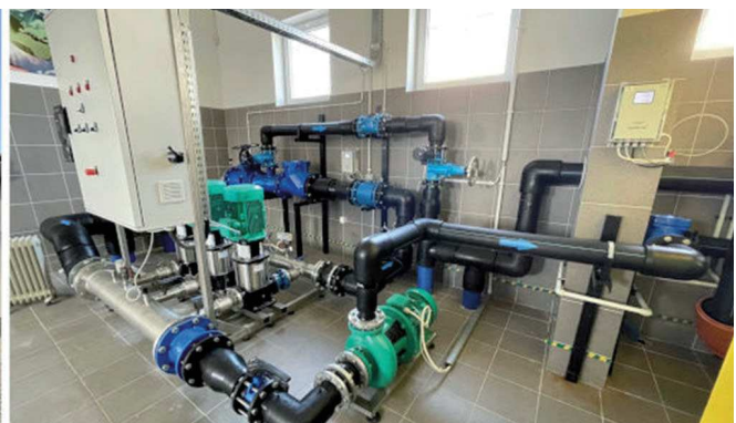
SUW Zamienie – zestawy pompowe
