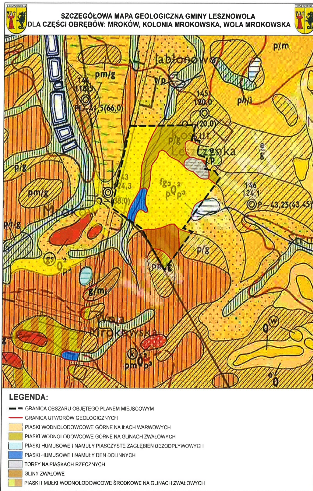
Rys. Podział geologiczny gminy według szczegółowej mapy geologicznej Polski.
