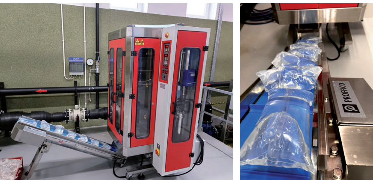
Konfekcjonowanie wody pitnej – paczkowarka
