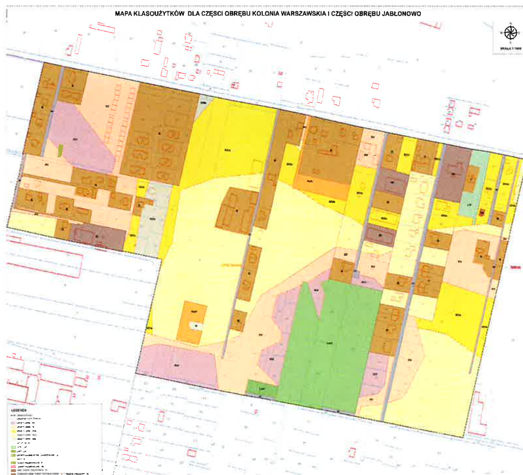
Rys. Podział obrębu Kolonia Warszawska na klasoużytki zgodnie z Ewidencją gruntów i budynków
