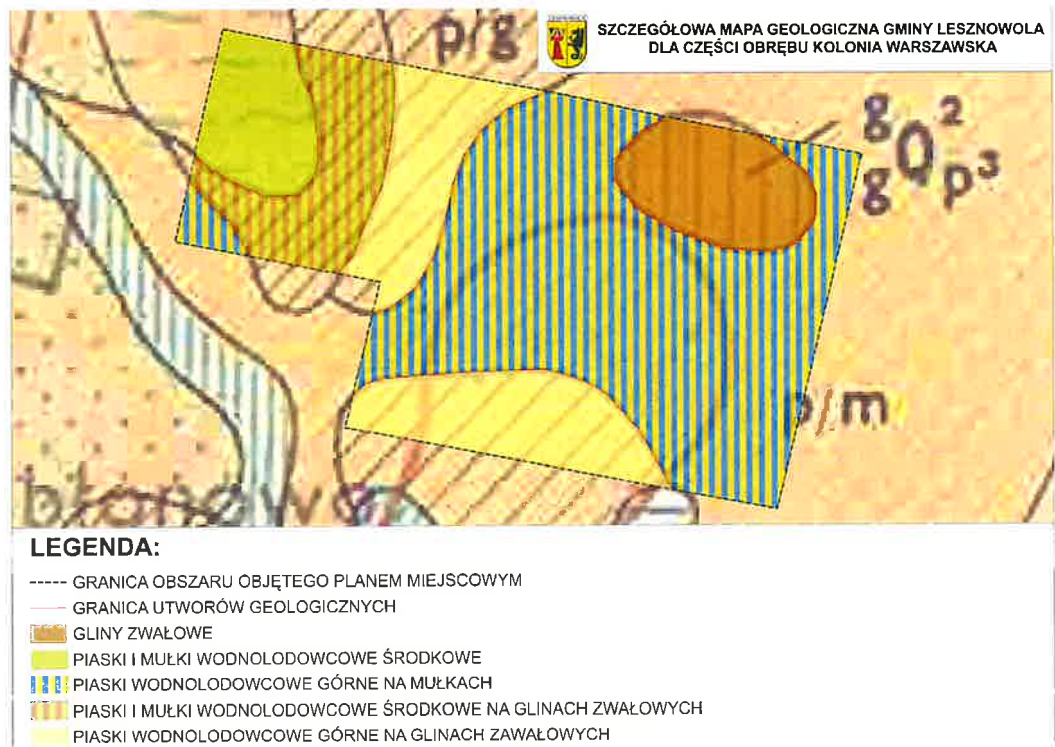
Rys. Podział geologiczny według szczegółowej mapy geologicznej Polski.
