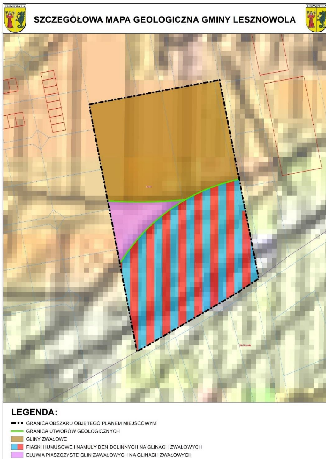
Rys. Podział geologiczny gminy według szczegółowej mapy geologicznej Polski – szczegółowa mapa
