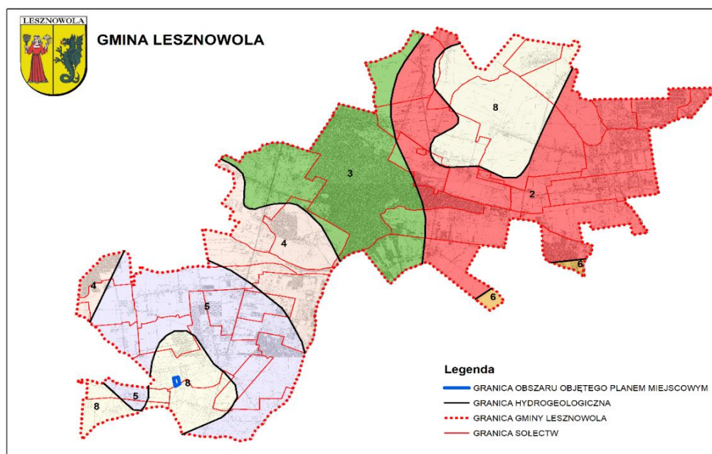
Rys. Podział hydrogeologiczny gminy Lesznowola według Mapy hydrogeologicznej Polski.
