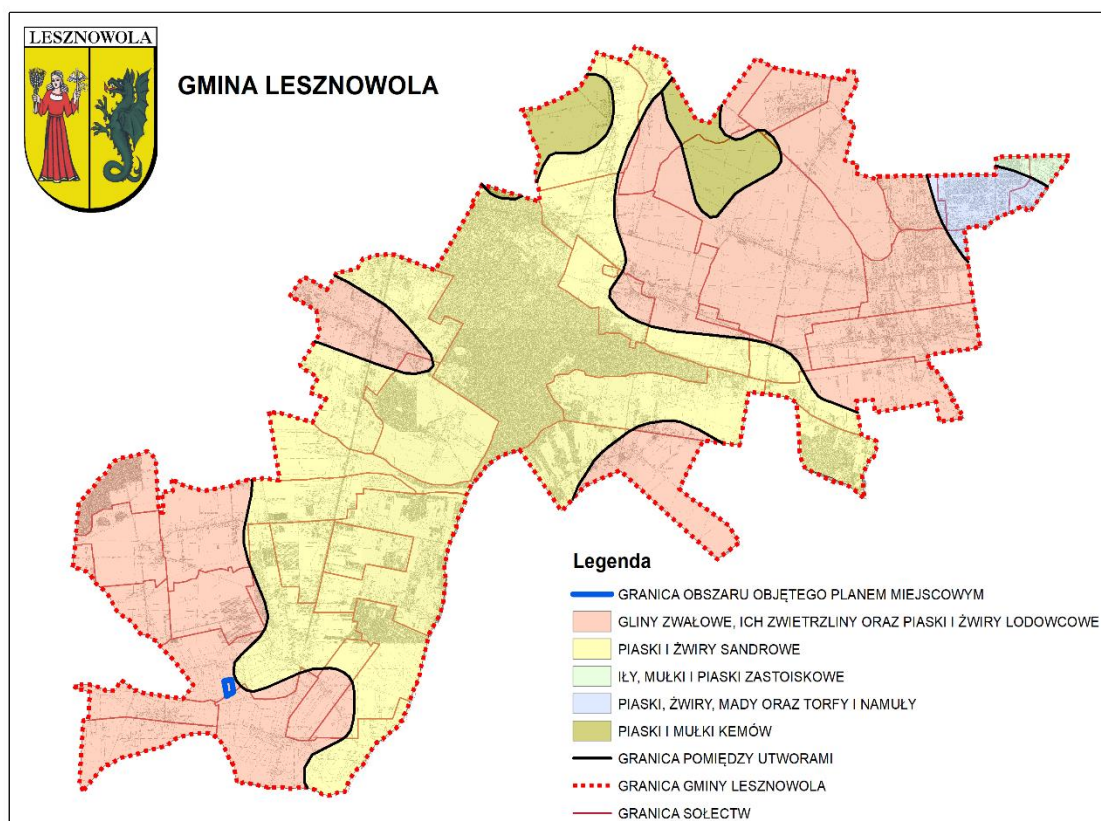
Rys. Podział geologiczny gminy według szczegółowej mapy geologicznej Polski.
