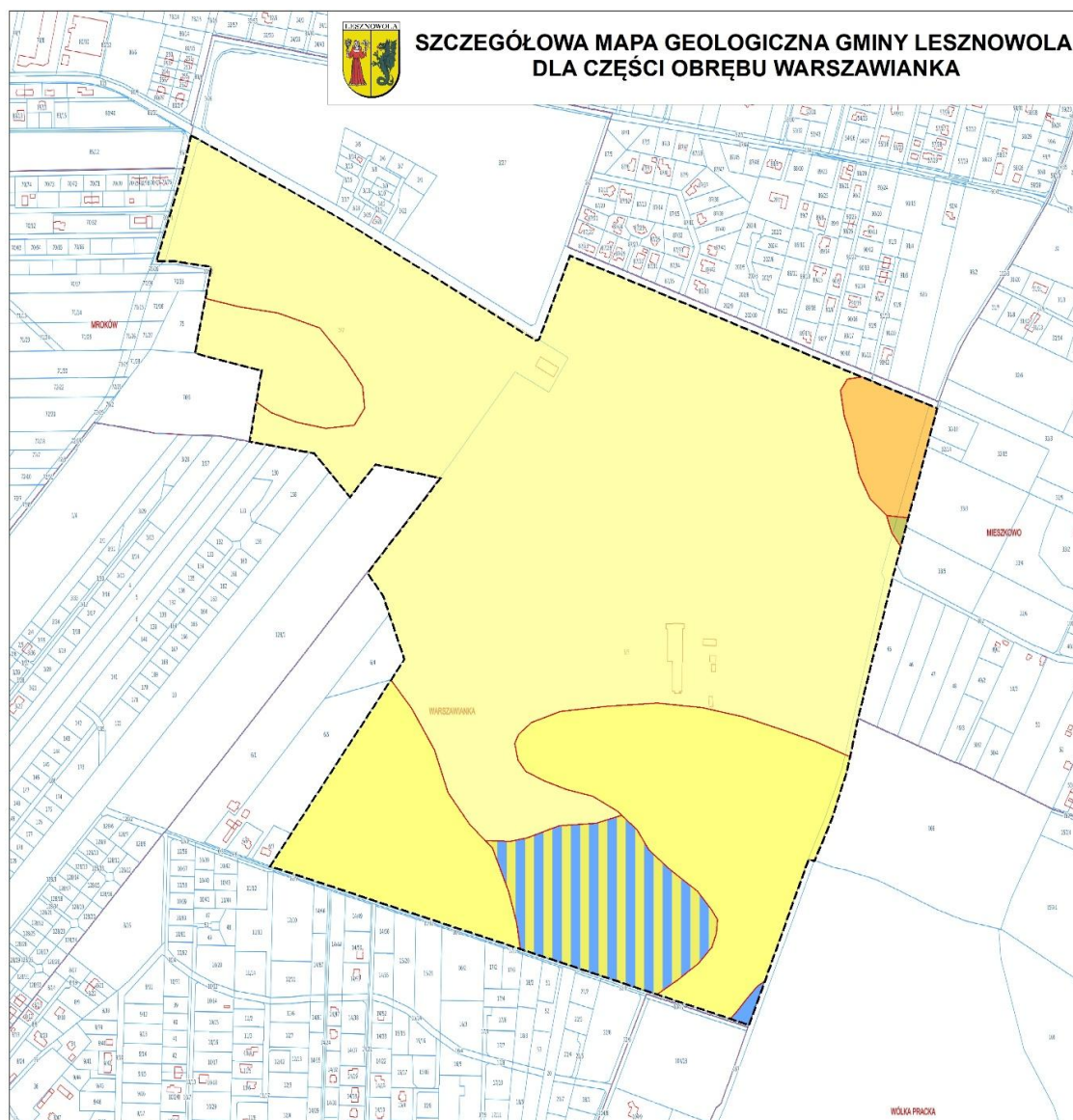
Rys. Podział geologiczny gminy według szczegółowej mapy geologicznej Polski.
