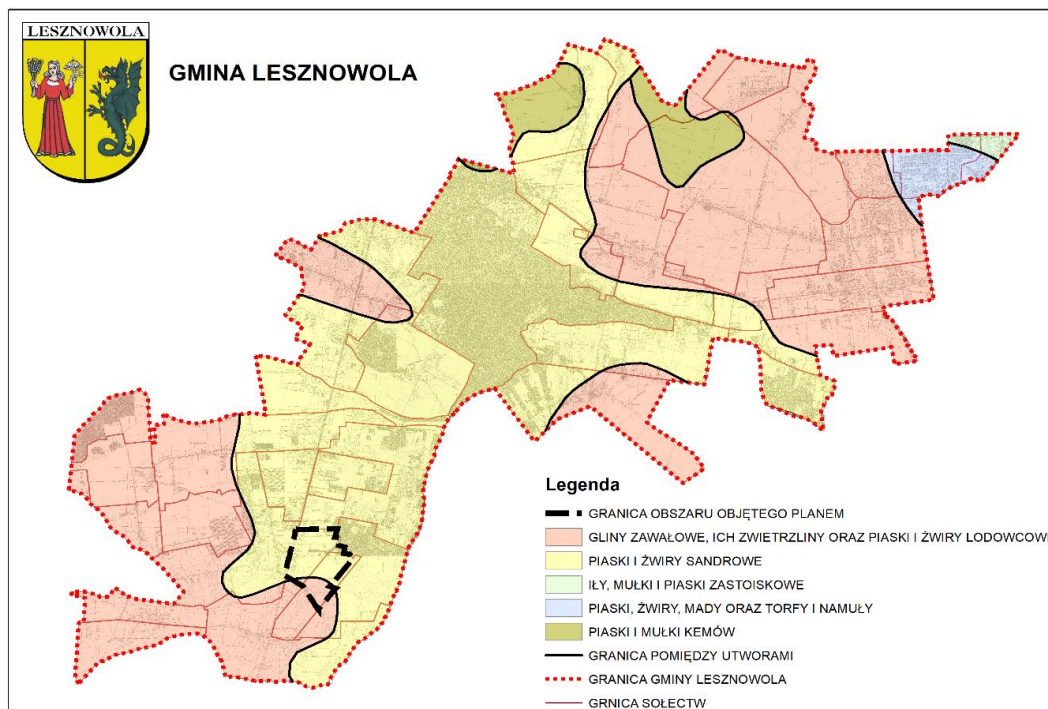
Rys. Podział geologiczny gminy Lesznowola według mapy geologicznej Polski.
