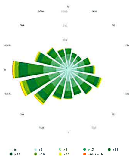
Rys. Róża wiatrów dla powiatu piaseczyńskiego w ciągu roku.
